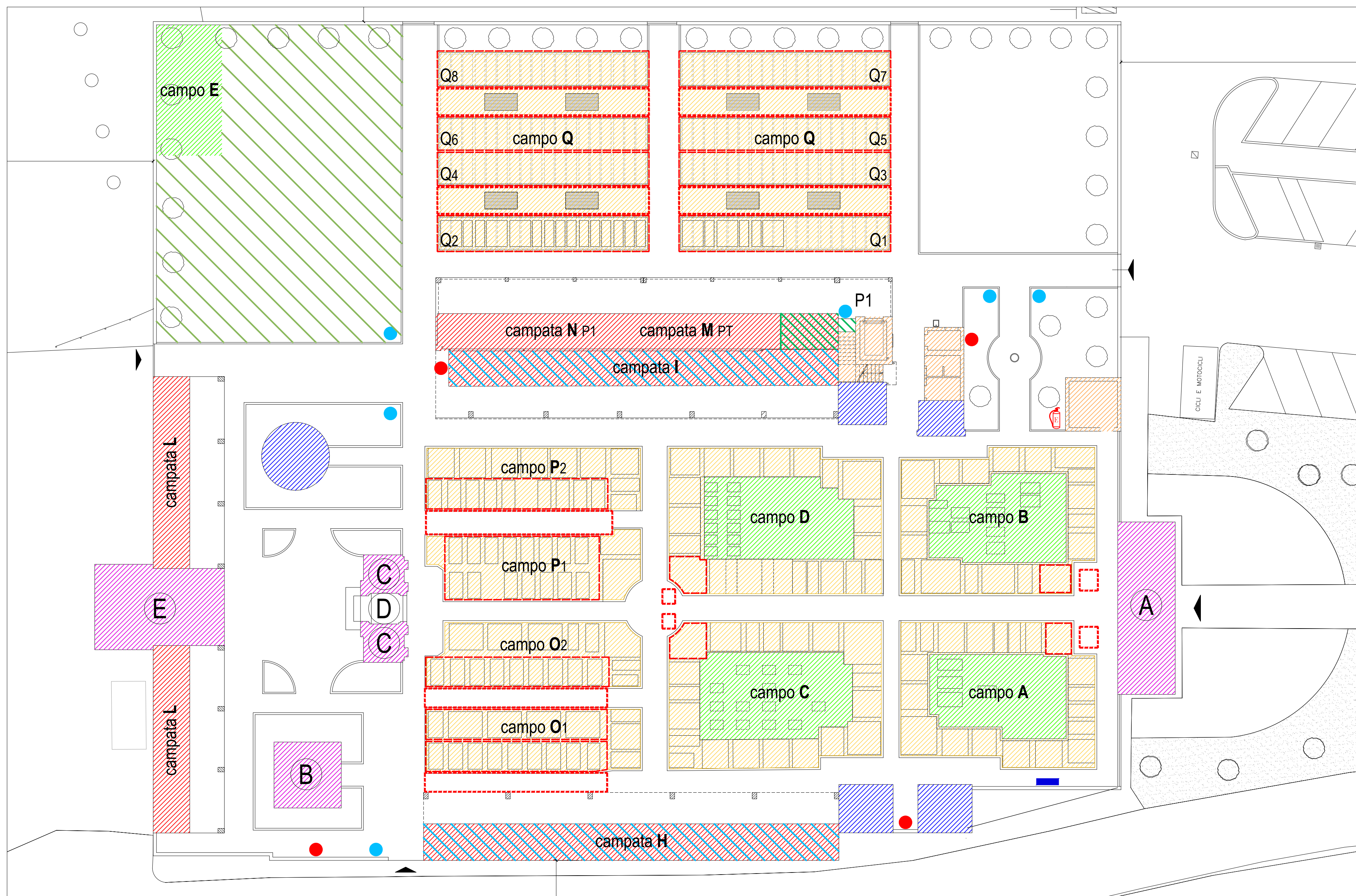
PLANIMETRIA GENERALE DELLO STATO DI FATTO scala 1:200
