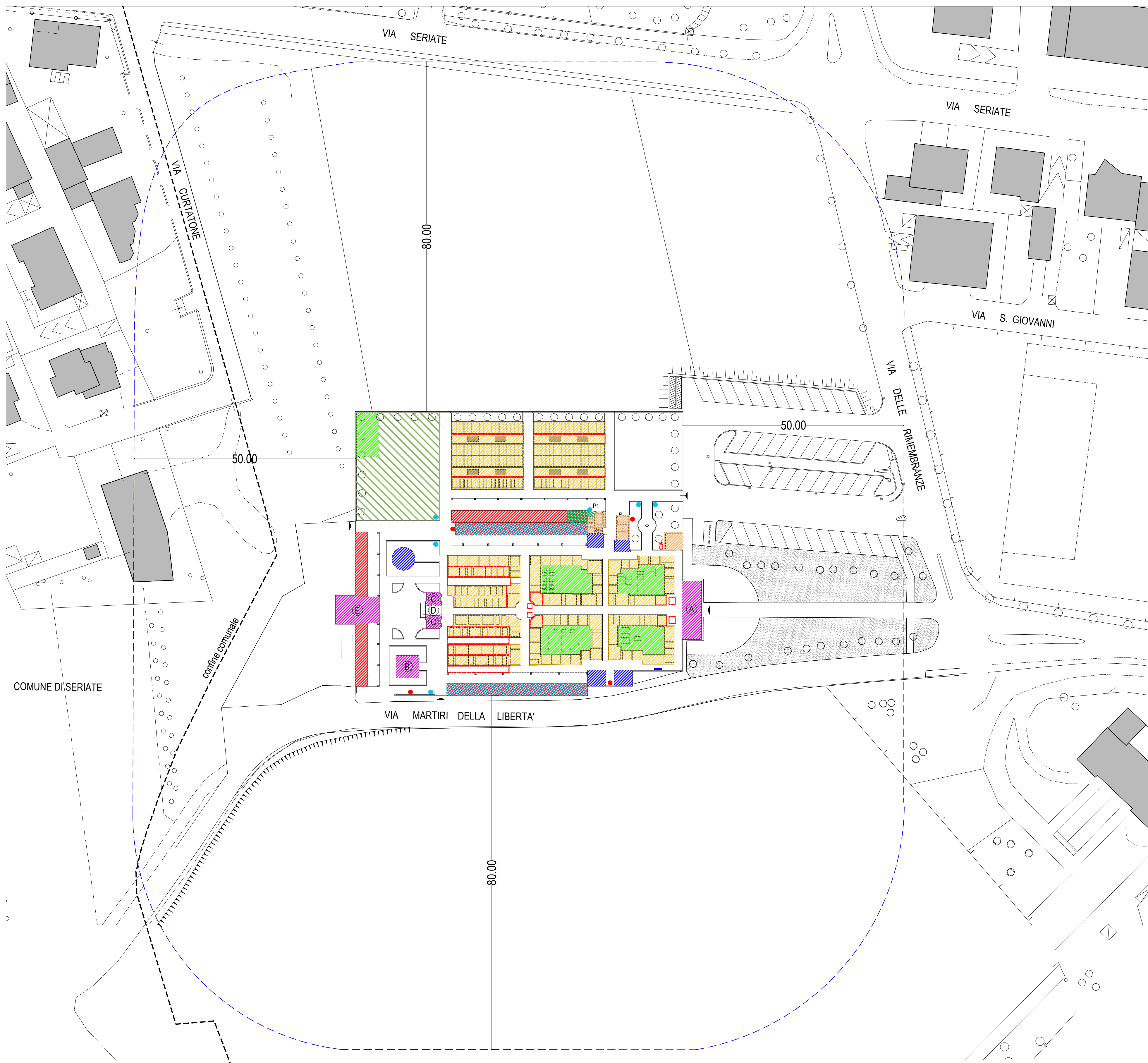
PLANIMETRIA GENERALE DELLO STATO DI FATTO scala 1:500
